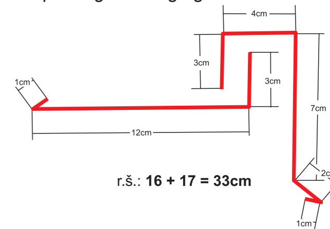
Lemovanie štítové dvojdielné vrchné Two-piece gable top edging
