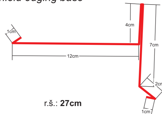
Lemovanie štítové základné Shield edging base
