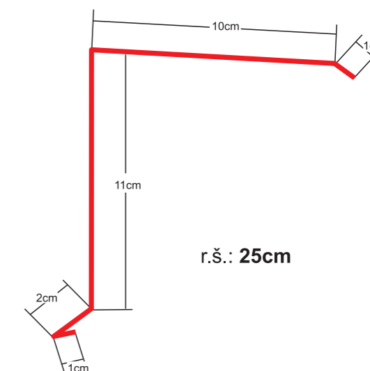
Lemovanie pultové základné Base counter edging
