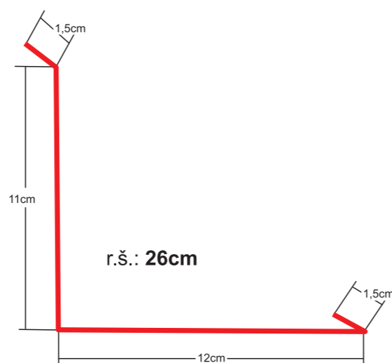
Lemovanie muriva bočné spodné Lining masonry side bottom
