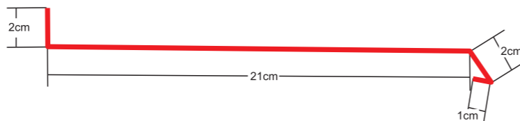
Parapet základný Basic window sill
