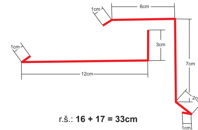
Lemovanie pultové základné Base counter edging
